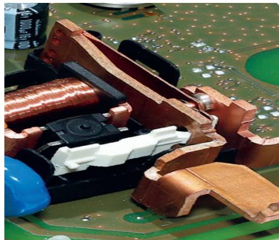
Le disjoncteur intégré au compteur Linky
