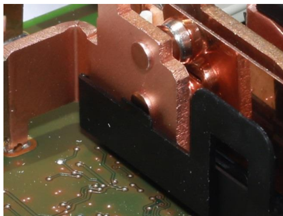
Détail du contacteur de puissance unipolaire du disjoncteur Linky
